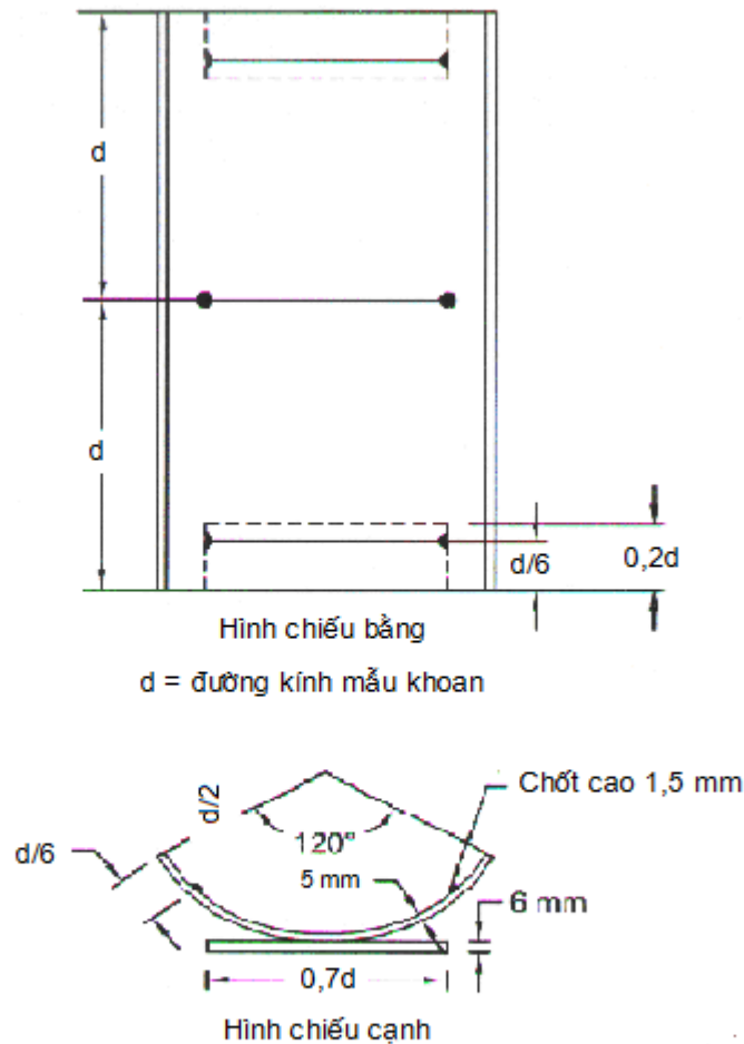
Hình 1 - dụng cụ thích hợp để làm phẳng mẫu khoan trong thí nghiệm xác định cường độ chịu nén khi bở
