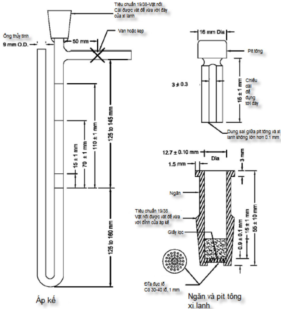
Hình 1 – Thiết bị thấm khí Blaine
