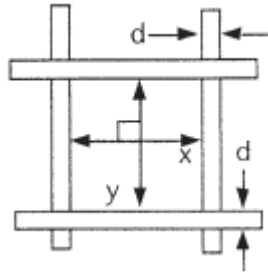
Hình 1. Kích thước thích hợp của ô lưới thép
